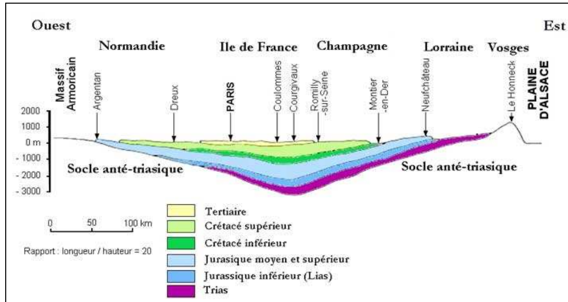
Figure 3 : Coupe géologique de principe du bassin parisien (Source : Burgéap 2008)
